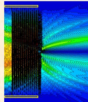
ミリ波渦場シミュレーション
