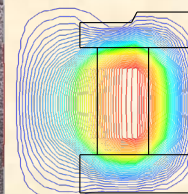
インダクター形状最適化
