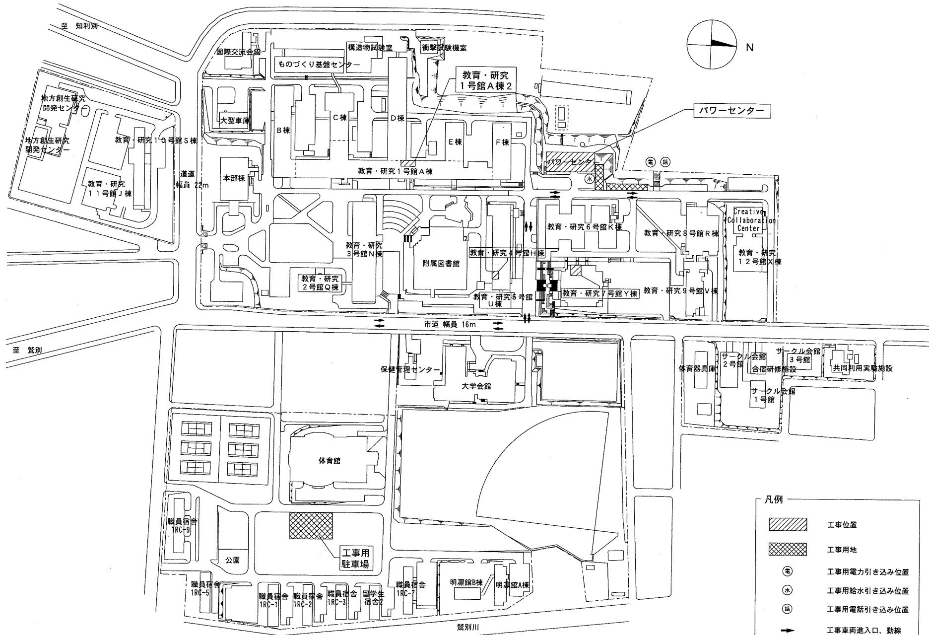
配置図 S=1/3,000
